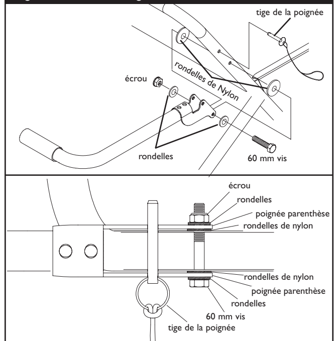
Figure 17 — Fixer la Poignée
